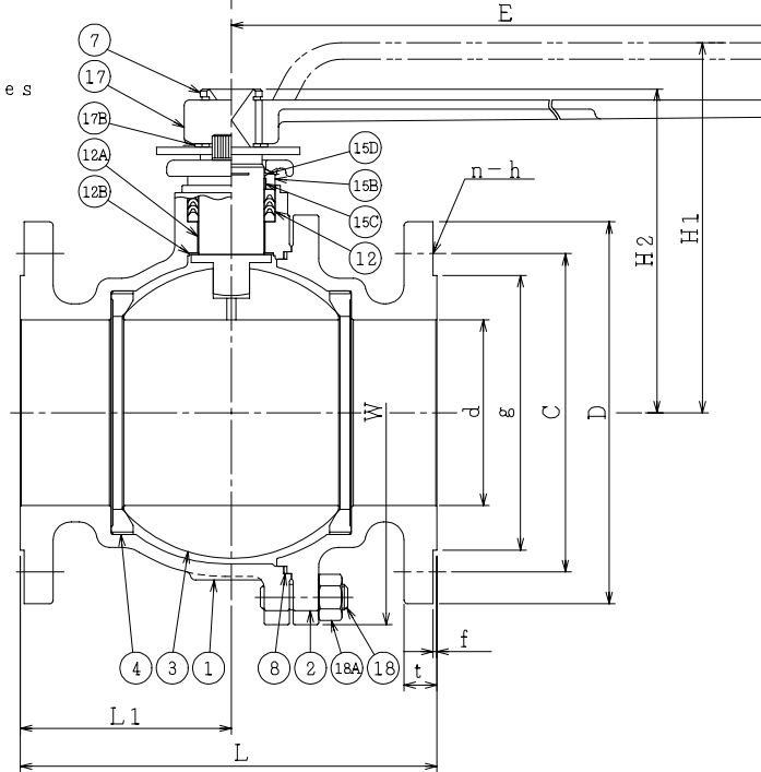
シート部詳細 Detail of Seat
