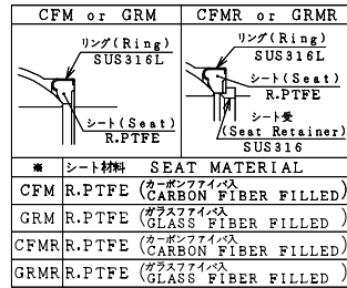
シート部詳細 Detail of Seat
