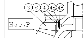
VSR4107NC-CF ソフト シート SOFT SEAT
