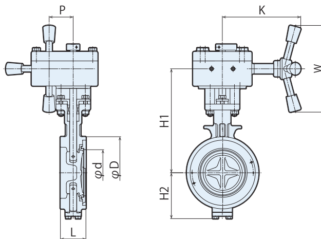
[ギヤ操作:KMG200形]
